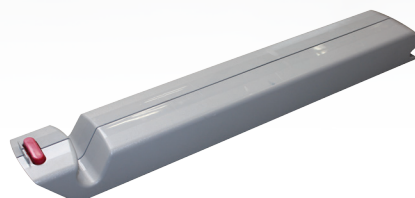
MBU0100 PB-Akku (Zellentausch/Reparaturauftrag) für ARJO Patientenlifter NDA0100-03/NDA0100-20 Marisa/Sara 3000 , 24,0V/4,0Ah
