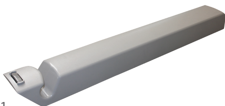
MBU0101 PB-Akku (Zellentausch/Reparaturauftrag) für ARJO Patientenlifter Tempo Opera Typ KPA0100-0510 , 24,0V/5,0Ah
